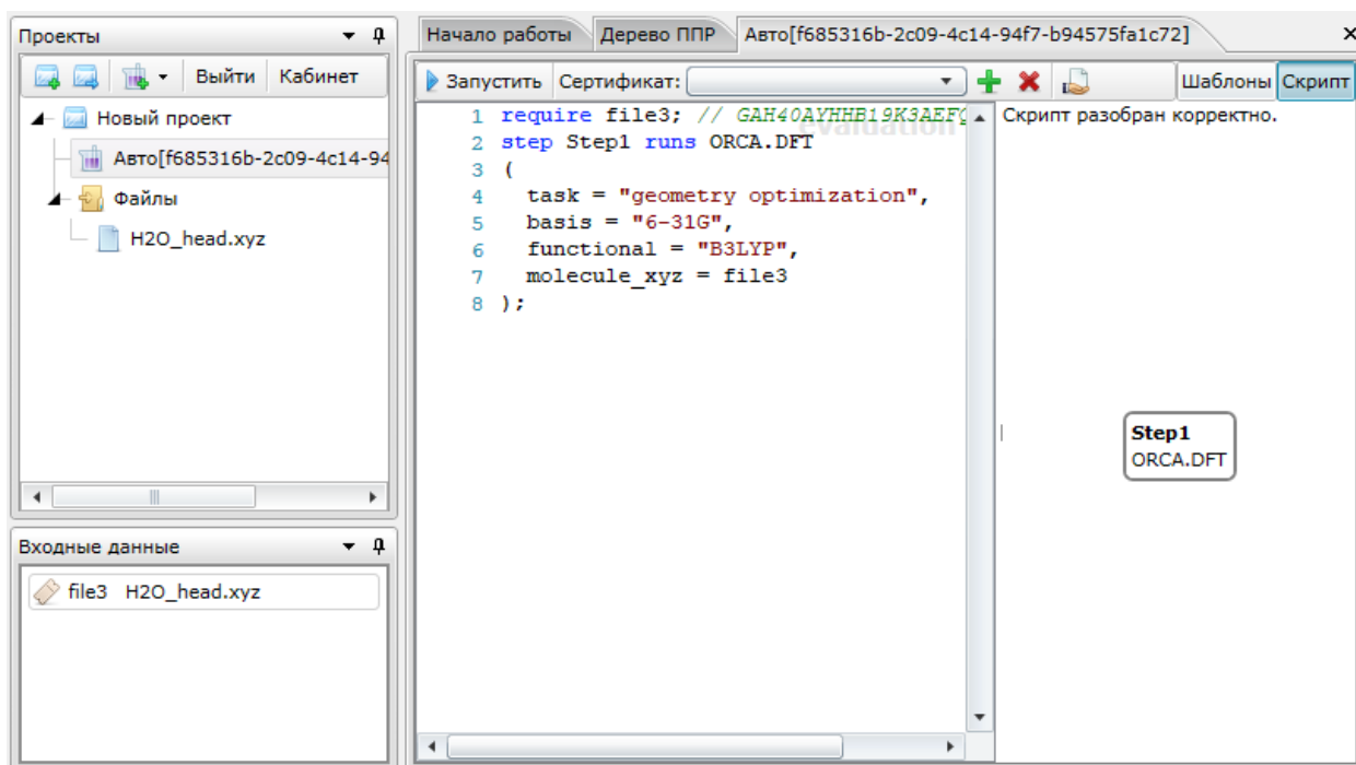
Рис. 3.10. Вид окна после опроса интеллектуальной системы
