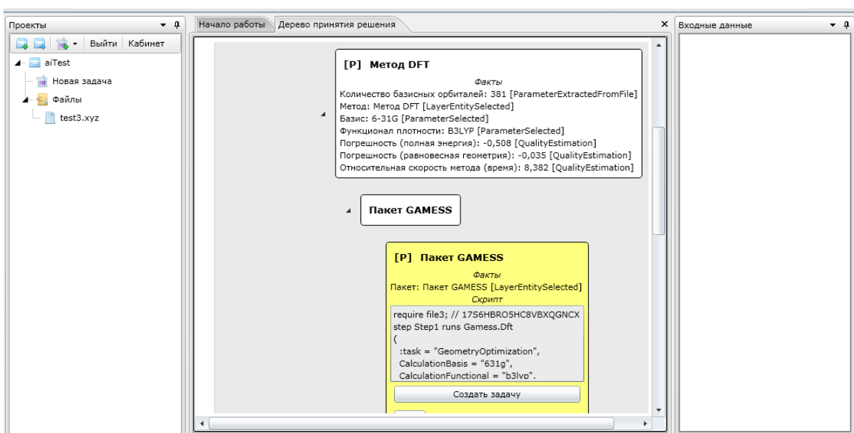
Рисунок 3.16 – Работа с деревом принятия решений
