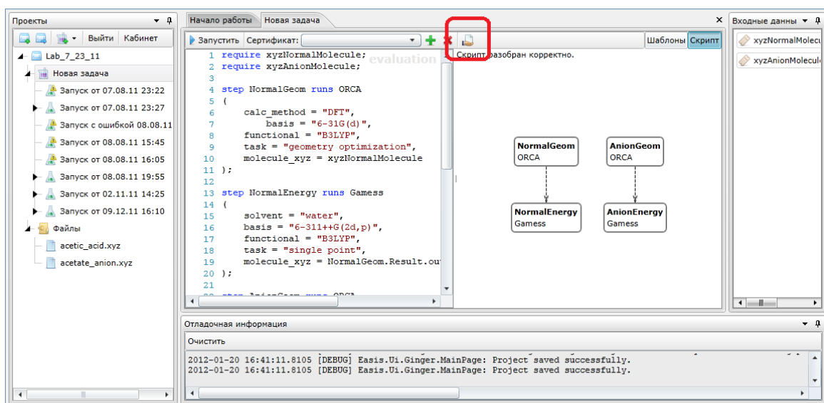
Рисунок 3.17 – Вызов публикации композитного приложения
