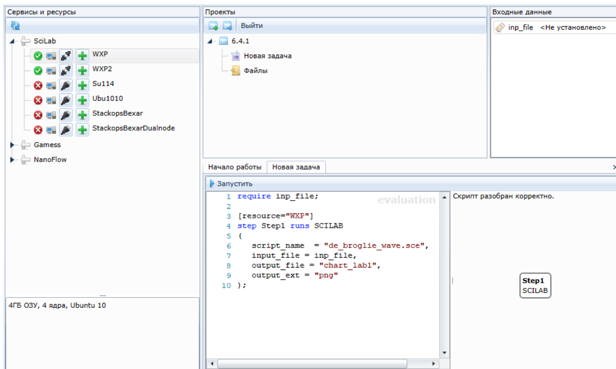
Рисунок 3.16 – Вид web-интерфейса после создания проекта и задачи
