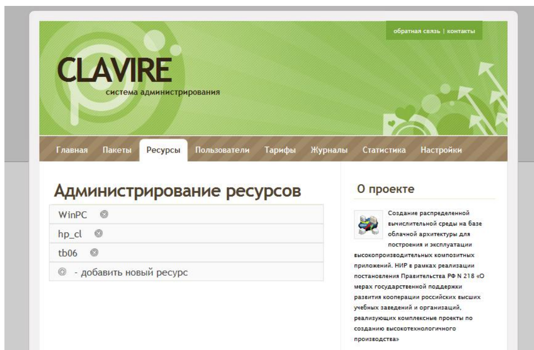
Рисунок 3.6 – Вкладка «Ресурсы»
