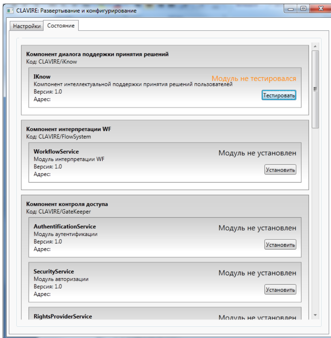
Рисунок 3.1 – Установленный модуль
