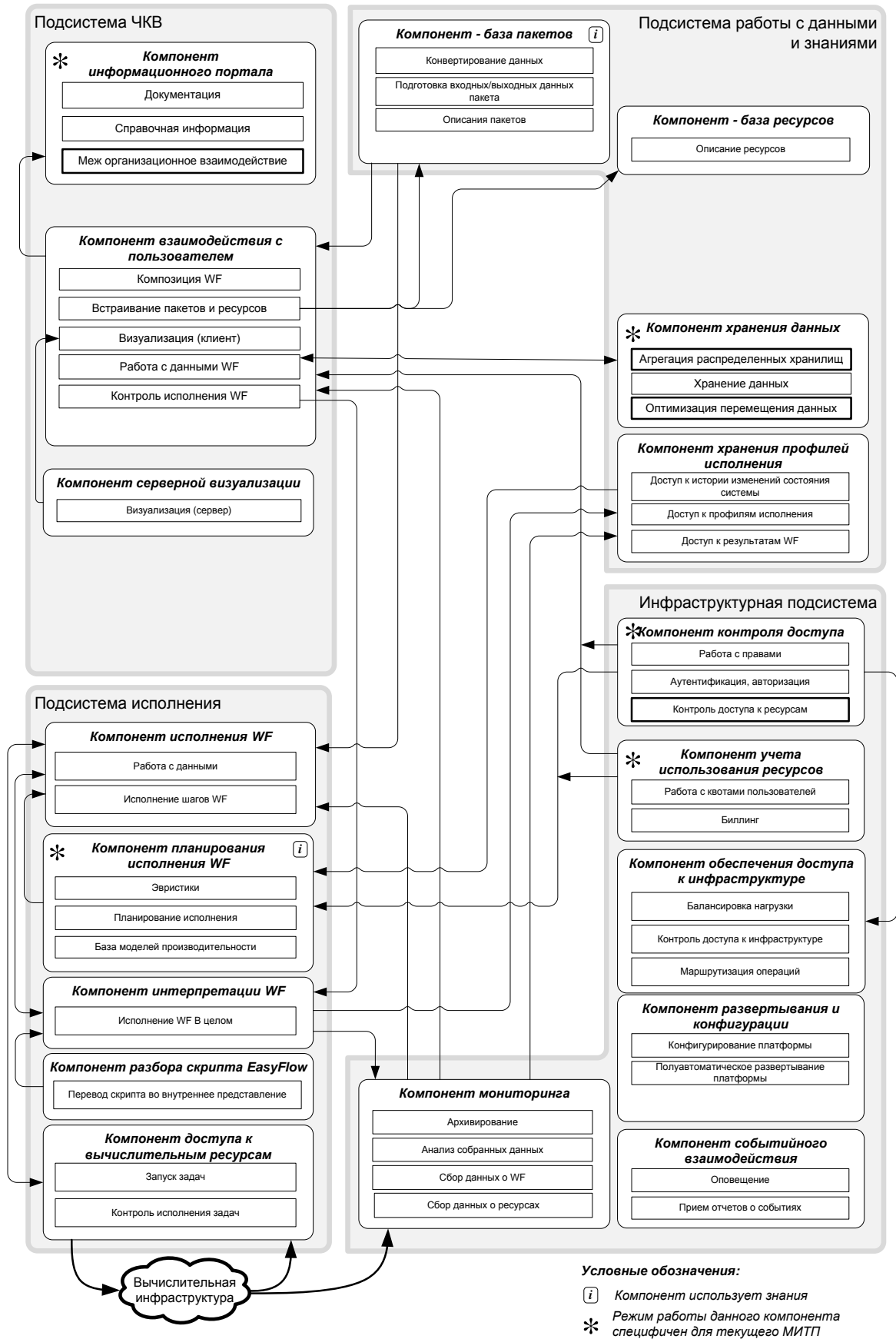
Рисунок 2.1 – Структура МИТП-М
